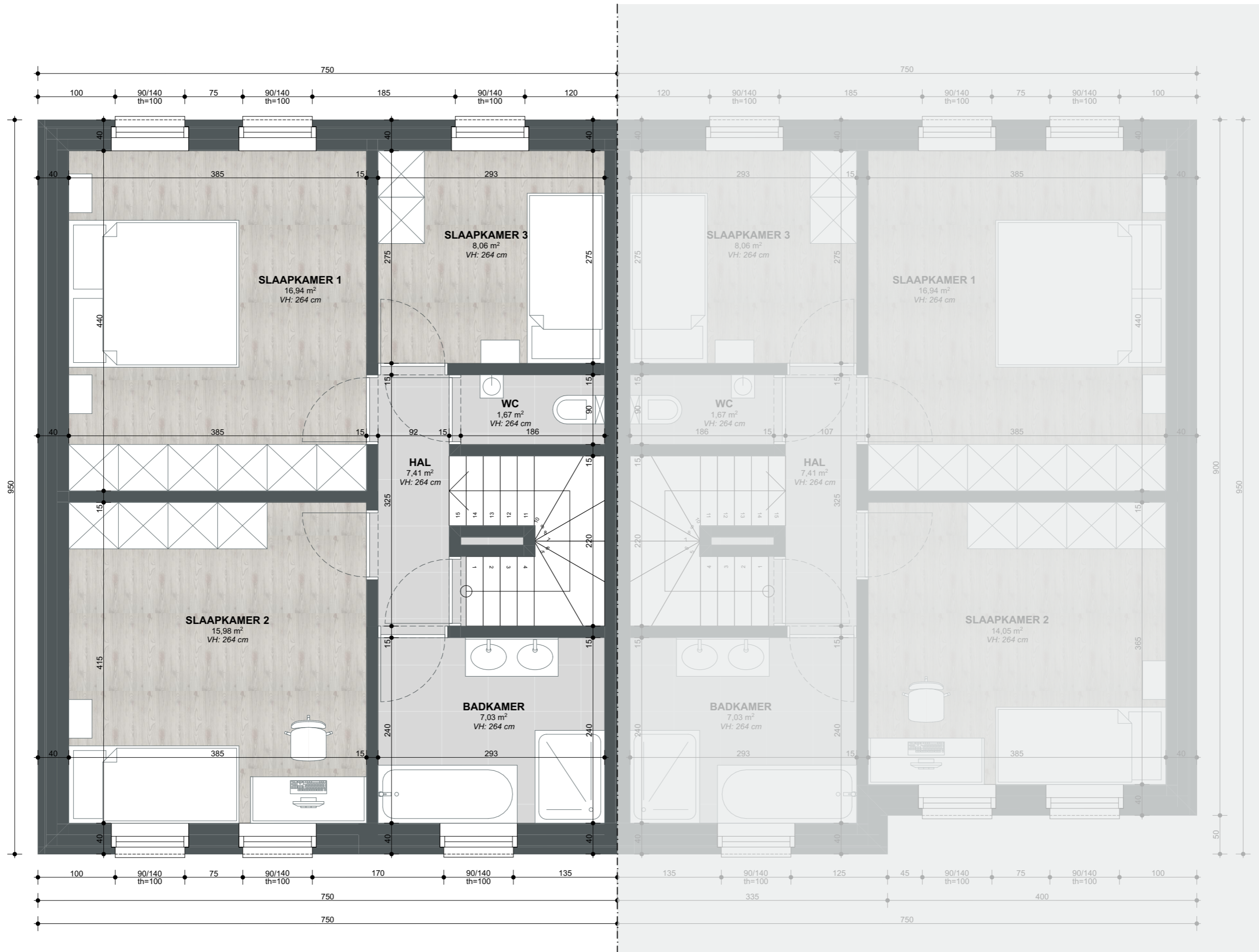
verdiepingsplan LOT 3 schaal 1/50
