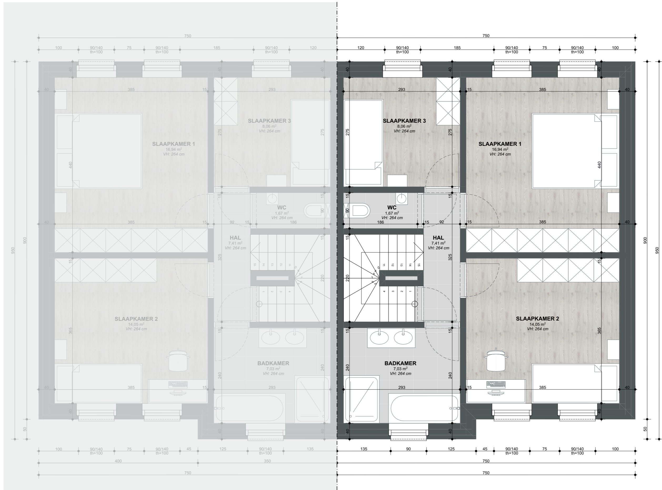
verdiepingsplan LOT 4 schaal 1/50
