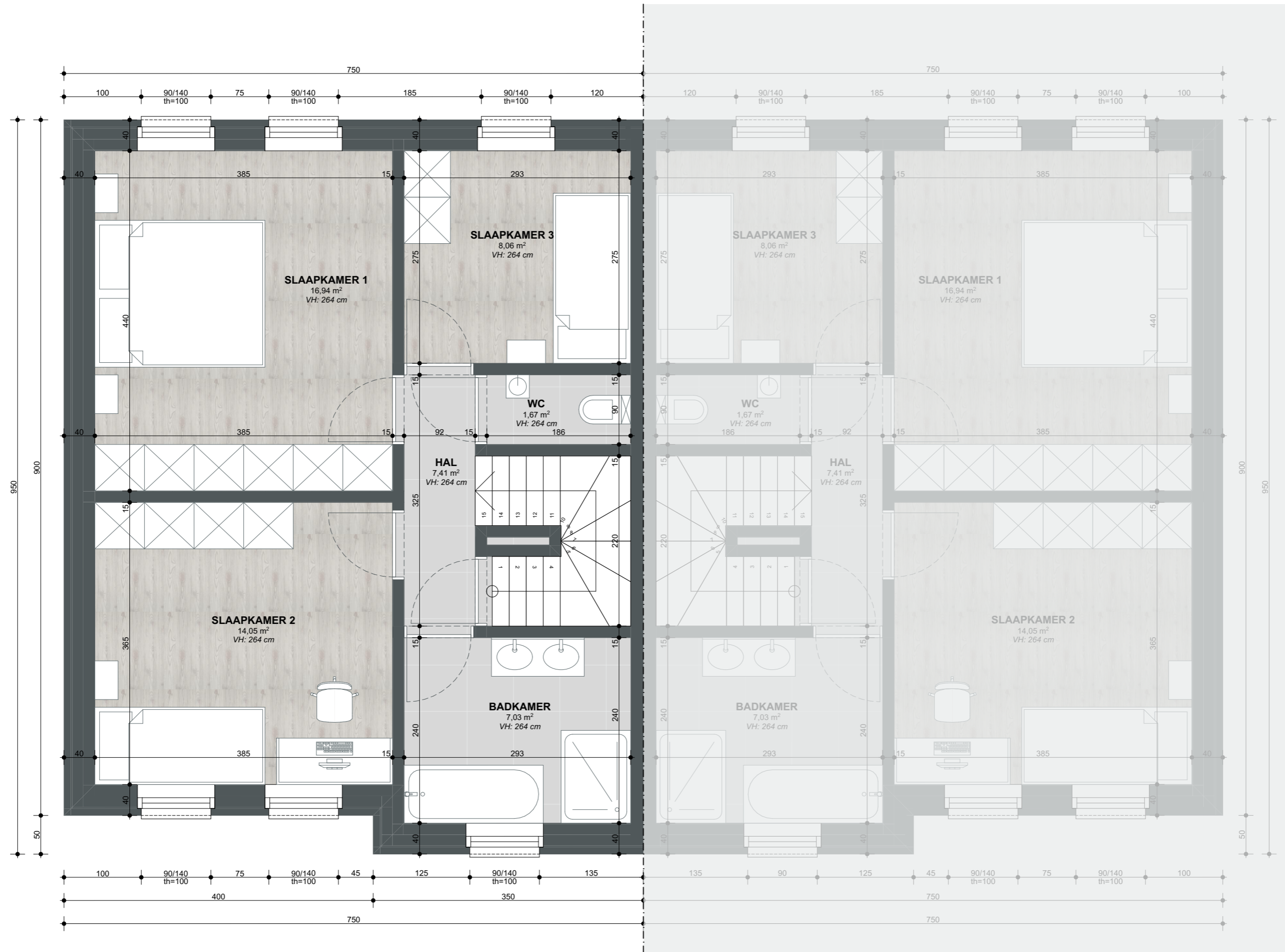
verdiepingsplan LOT 5 schaal 1/50
